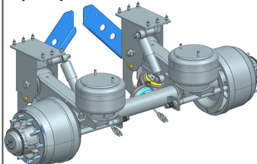
Suspensão para chassi modular
